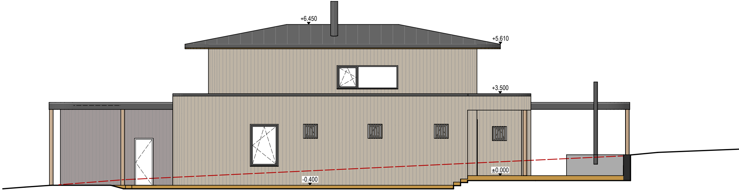
POHLED SEVEROZÁPADNÍ
