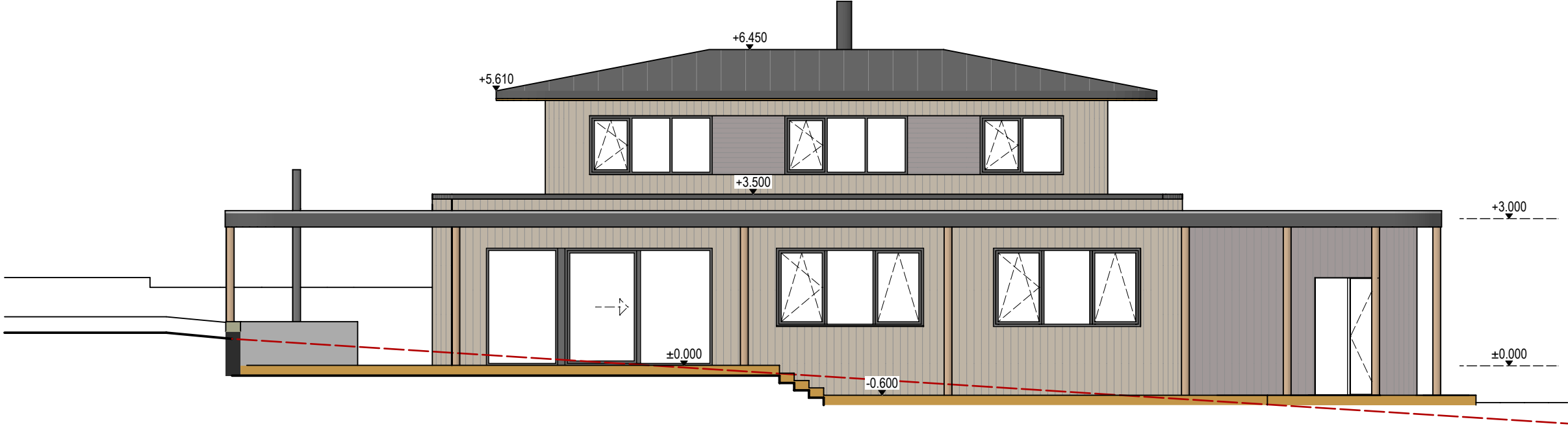
POHLED JIHOVÝCHODNÍ
